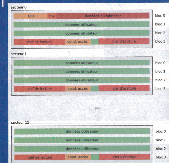
Figure 3 : Structure de la mémoire d'une Mifare Classic 1K
