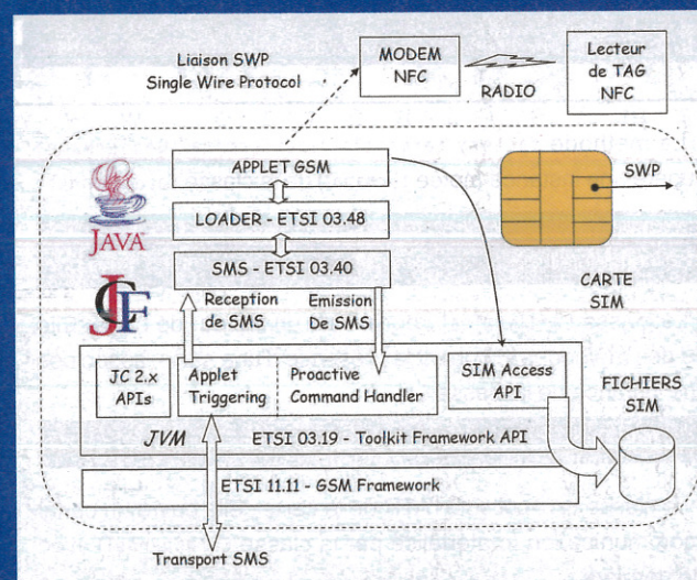
8 Écosystème de la carte SIM
