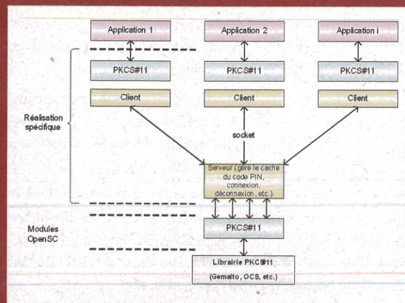
3 Architecture d'une solution de gestion de cache du code PIN
