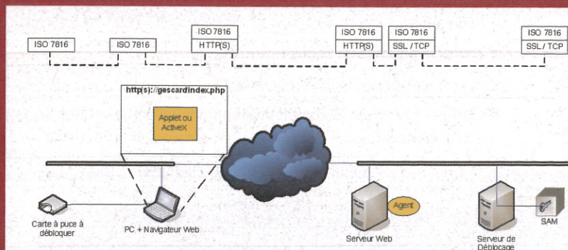
2 Architecture d'une solution de déblocage
