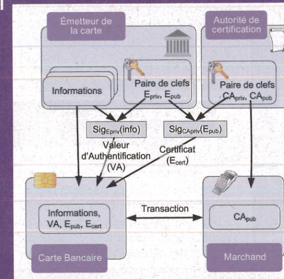
2 Organisation des acteurs dans le protocole de paiement EMV avec SDA
