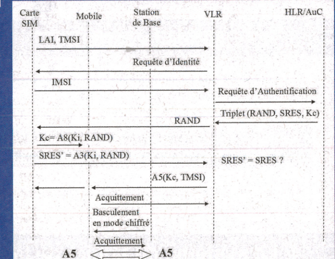
2 Principes de sécurité d'un réseau GSM
