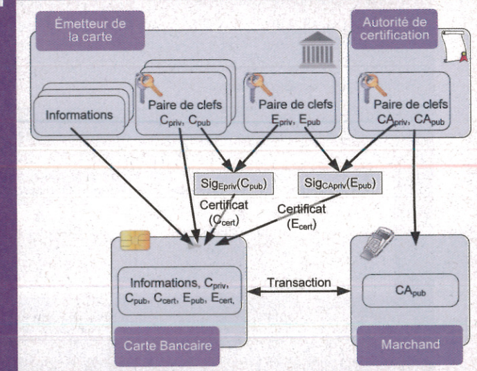
3 Organisation des acteurs dans le protocole de paiement EMV avec DDA
