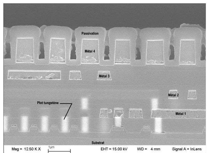
Vue en coupe
