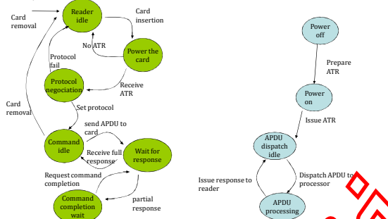
Diagramme d'état du lecteur
